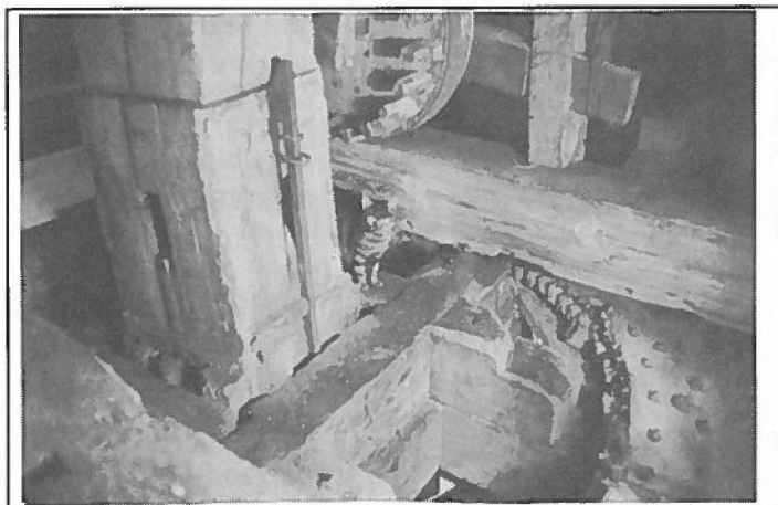
Foto vanaf de luizolder van "De Jonge Hendrik" De oude standaard uit Niekerk werd na 1847 koningspil. De uiteinden van de kruisarmen zijn duidelijk uitgespaard voor de acht plooiestukken van het standerdmolen-bovenwiel. (foto: MEVD, 11 oktober 1994)
