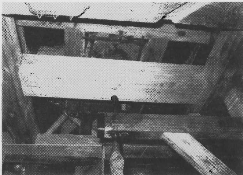
De nieuwe eiken taatsbalk na plaatsing in de steenzolder. Rechtsonder de steenkraan. De steenzolder is daar vrij laag, vandaar de sleuf in de legeringsbalk uiterst rechtsboven voor de schroefspindel. Opname naar het noorden gezien.
