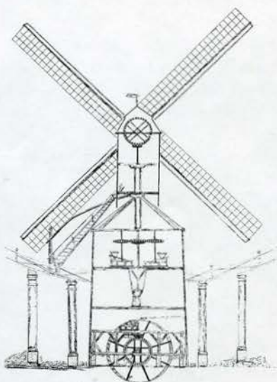
Bouwaanvraag voor een windmolen te Kruishoutem op een reeds bestaande korenwatermolen, 1854.
