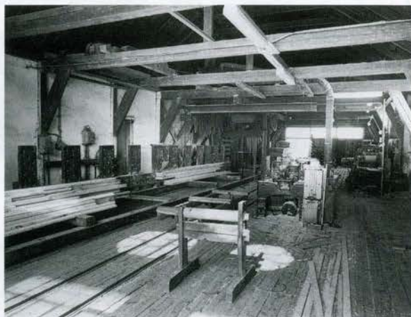
Interieur van de zaagloods, gezien naar het zuiden (afvoerszijde); links het elektrische battingraam, rechts het grote zaagraam met de slede.
