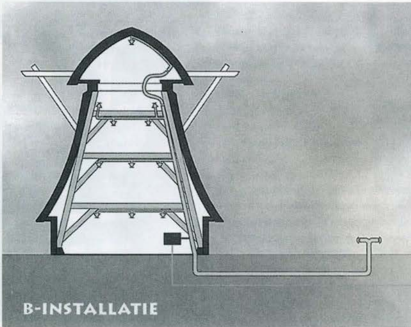
Semi-automatische sprinklerinstallatie ( Info , 2000-20, Rijksdienst Monumentenzorg)
