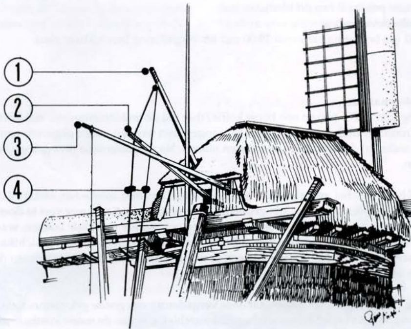
Zwichtbomen achter op de kap: bezaanstk (1), zwichtboom (2), vangstk (3), zwichtketting (4)
