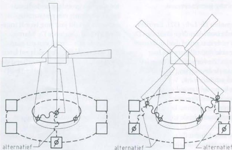
Aarding van windmolens (NEN 1014). (Let op de draairichting!)
