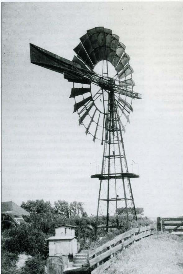
Eén van de door Loning gebouwde windmotoren, ± 1972 (Medemblik)
