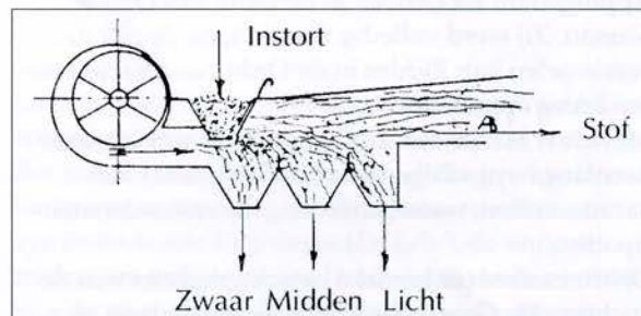
Schema wanmolen met druklucht
