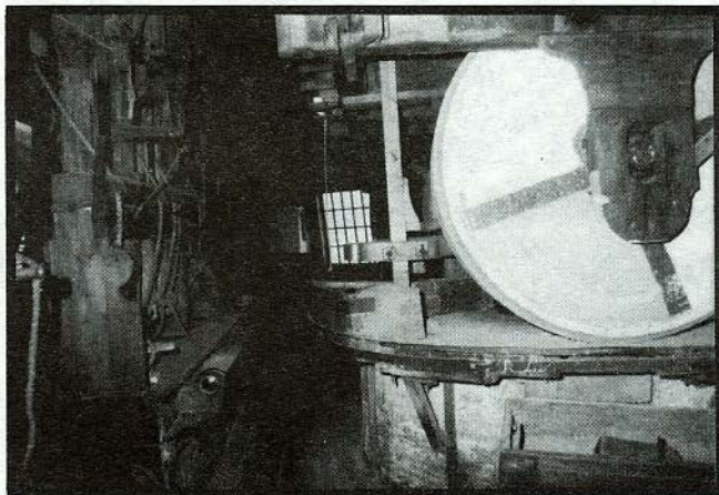
Interieur van een oliemolen. Links het naslagwerk en rechts de kollergang. De foto is weliswaar genomen in oliemolen "Het Pink" te Zaandam, maar het principe is vrijwel gelijk.
