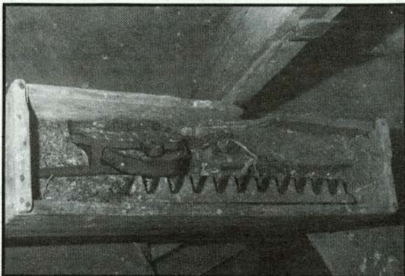
Herinnering aan de tijd dat de "Eva" een zelfkruier was: een stuk ringtandheugel en een keerschijf in de kist op de vangbalk.
