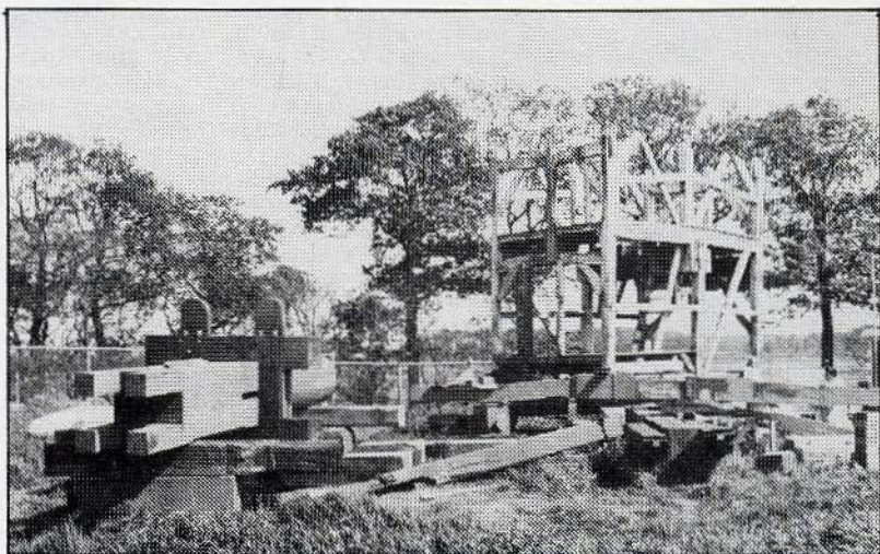
De zeer omvangrijke restauratie van de standerdmolen te Ter Haar. Links de nieuwe stander met onderzetel, rechts de ontmantelde oude kast met ervoor de kruisplaten. Foto 18 mei 1986.
