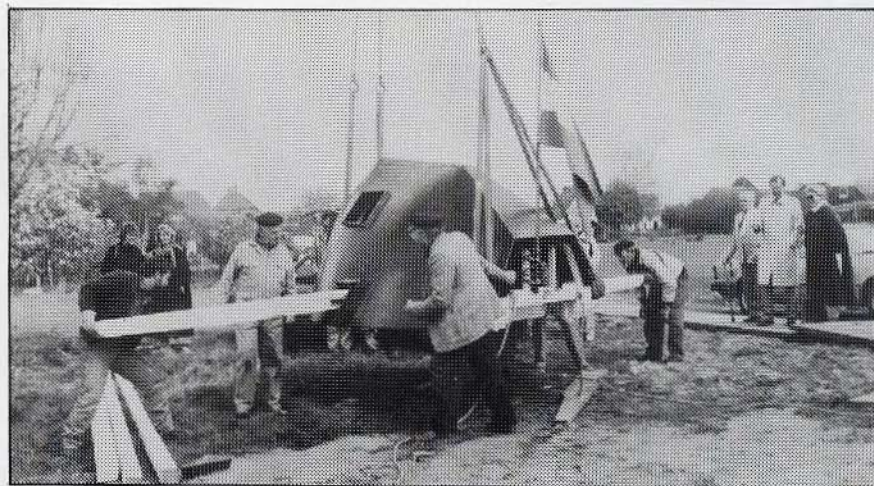
Vóór het ophijsen van de kap wordt de lange spruit nog even ingestoken. Duidelijk is het "manluik" links op de kap te zien.
