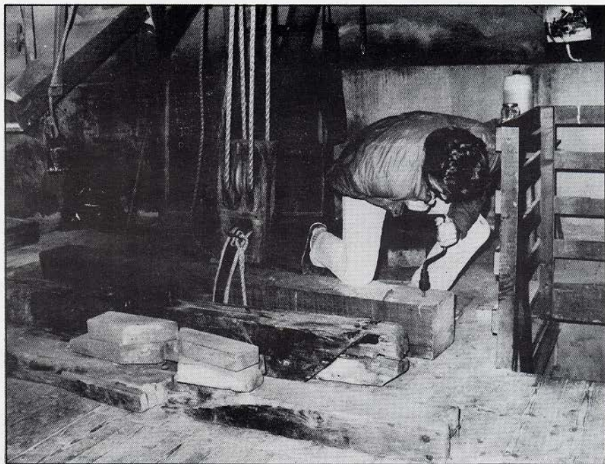
In de molen "De Lelie" te Eenrum is vrijwilliger Tom Baars hier aan 't werk met de nieuwe ijzerbalk. Op de voorgrond de oude, kapotte ijzerbalk en ervoor ligt de vermolnde achtkantveldregel, die de ijzerbalk droeg.
