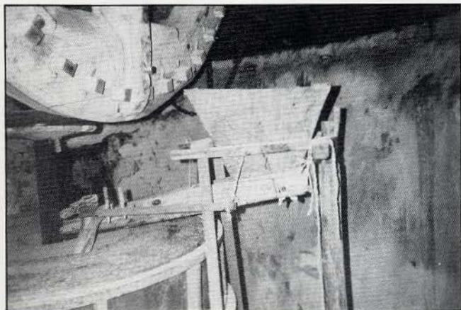
Kaar met schuddebak (schoe), die met een houten klos op de steen rust. Ook is een gedeelte van het bovenwiel (zonder vang!) zichtbaar.
