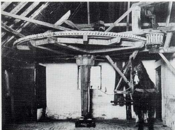
Een rosmolen in gebruik. Men ziet rechts het paard. In dit geval een afbeelding van een voormalige karnmolen van Jelle Hoekstra te Suameer (Friesland).
