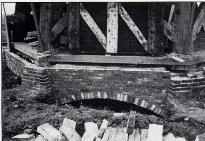
De "Zuidwendinger Watermolen" heeft een nieuwe fundering gekregen. Het achtkant is op de foto nog niet rechtgezet door het plaatsen van de peuthouten onder de achtkantstijlen.
