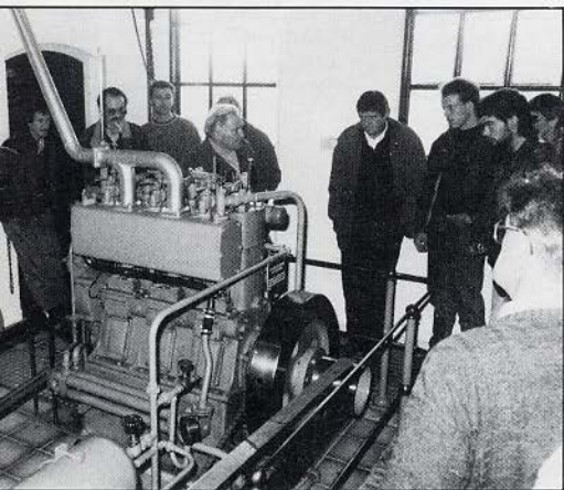
Dieselmachinist Kramer doet uitleg aan onze vrijwilligers in het gemaal "De Hoogte" te Nieuwolda. Op de foto de fraaie Brons-dieselmotor uit 1935.
