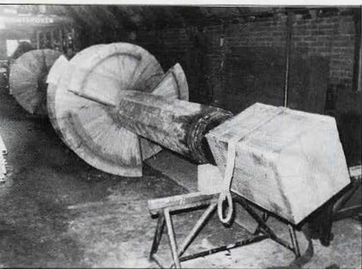
De kapotte vijzel van "De Krimstermolen" in de werkplaats van de molenmaker.
