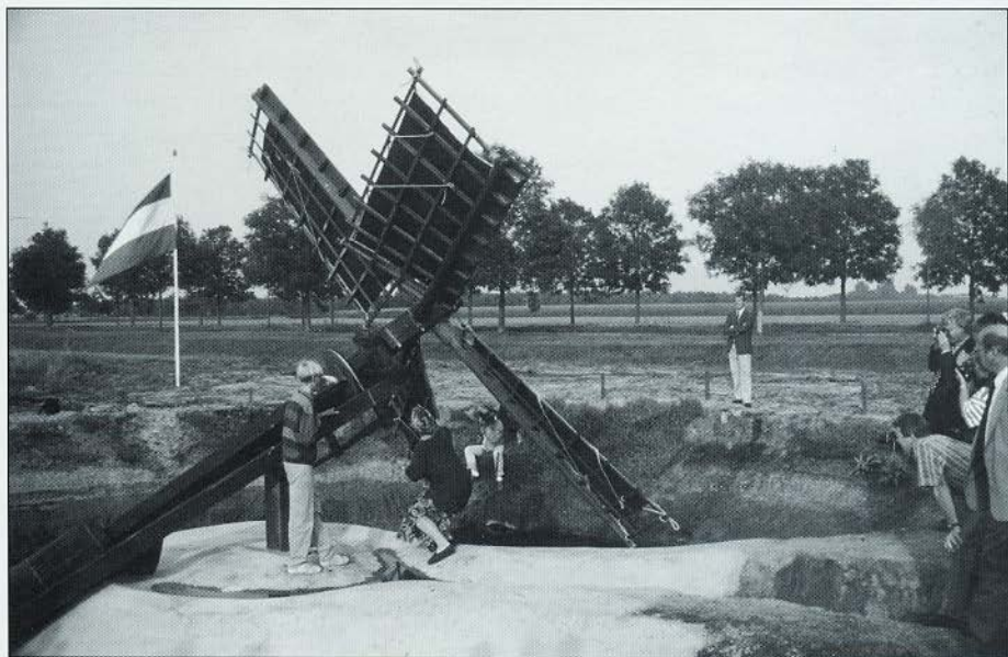
De feestelijke ingebruikname van de nieuwe tjasker in Midwolda. Foto: F.L. Humbert 20-9-1993.
