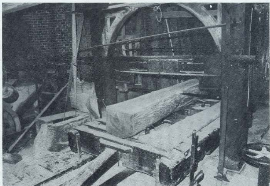
Aandrijfwerk van een zaagmaan met horizontale zagen. Een soortgelijk werktuig zagen we in de Rutteler Molen. (foto: MEvD)
