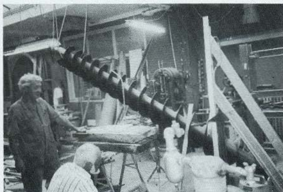
De vijzel in de werkplaats van de molenstichting (foto: T. Kalk, juli 1995)
