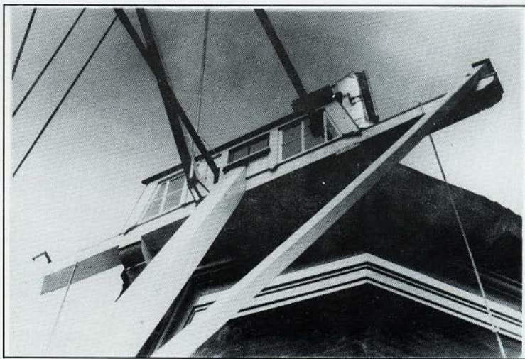
Het veranderde 'achterwerk' van de kap van de koren- en pelmolen DE JONGE HENDRIK
